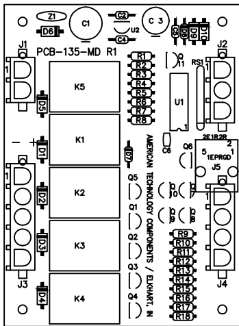
PCB-135-MD R1 -- ASSEMBLY
